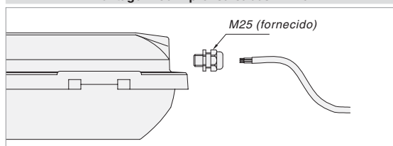
Montagem com prensa-cabos "E xe"
