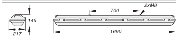
Luminária 58W - NA96372/NA 96373/NA 96383
