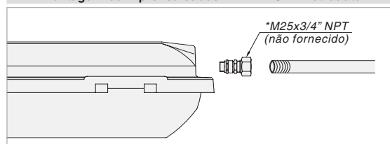
Montagem com prensa-cabos NEA2FRC + Eletroduto
