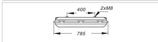
Luminária 18W - NA96547/NA 96548/NA 96518
