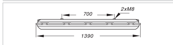
Luminária 36W - NA 96553/NA 96555/NA 96525
